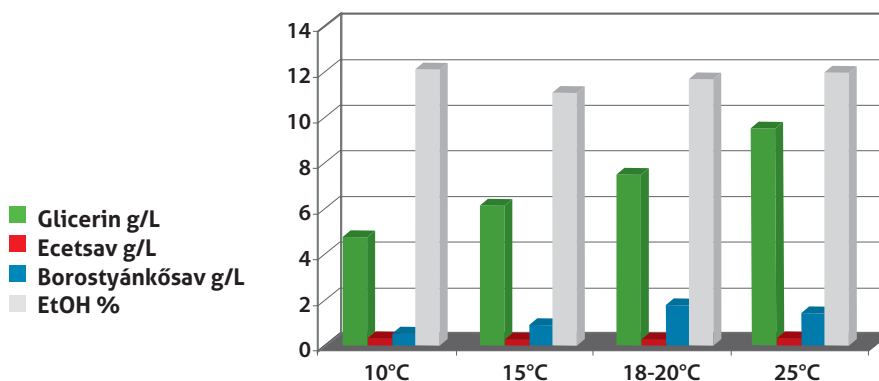
A hőmérséklet hatása a W15™-re
